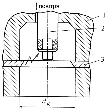
Рис. 1. Схема БРБ
