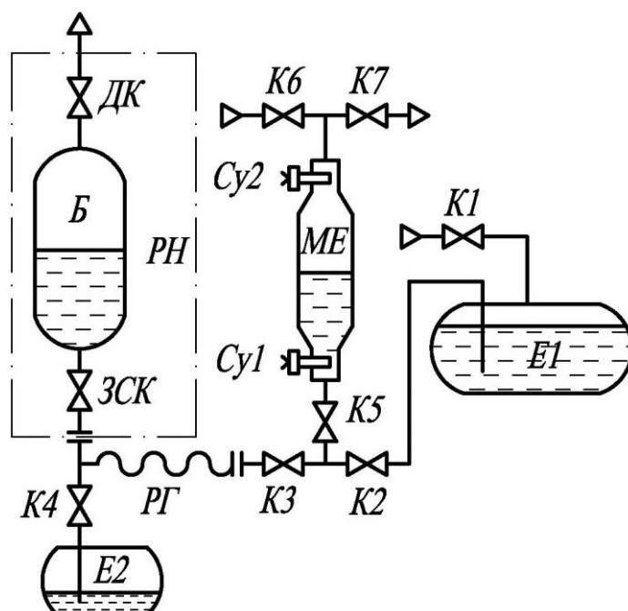
Рисунок 3 – Схема дозирования с применением мерной емкости:
