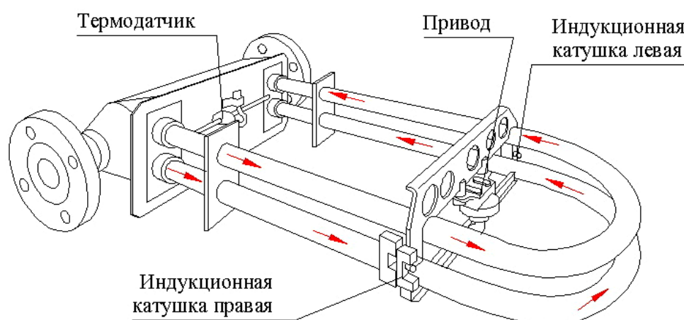
Рисунок 7 – Принцип действия массового расходомера Micro Motion
