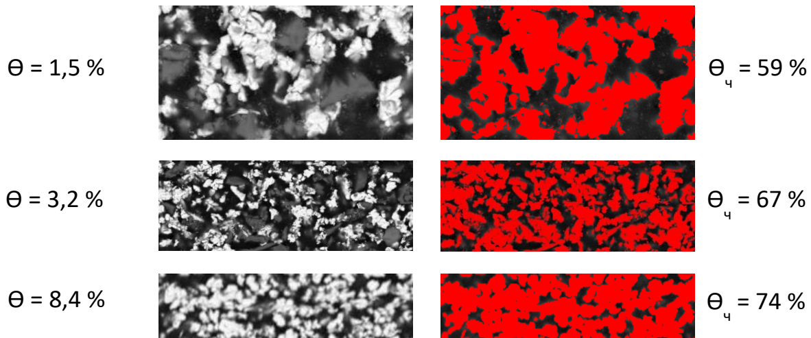
Рисунок 2 – Обробка зображень для визначення локального об'ємного вмісту частинок у струмопровідних шарах
