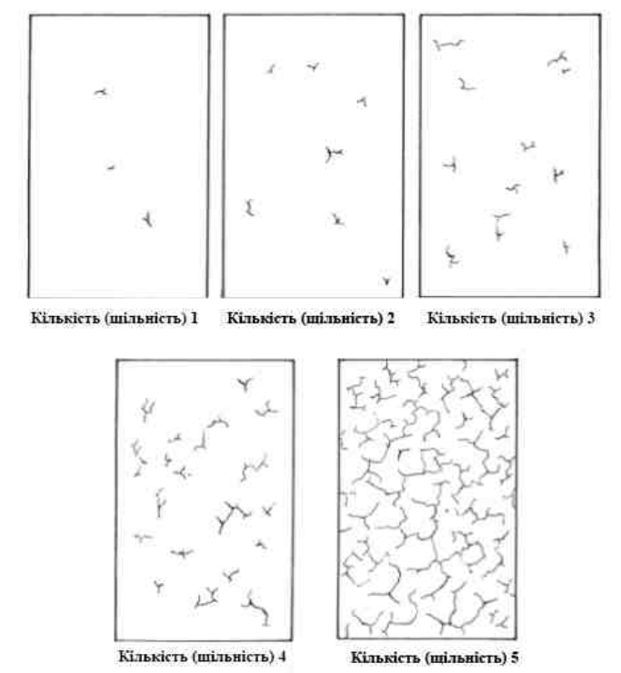
Рис.1. Розтріскування без виділеного напрямку
