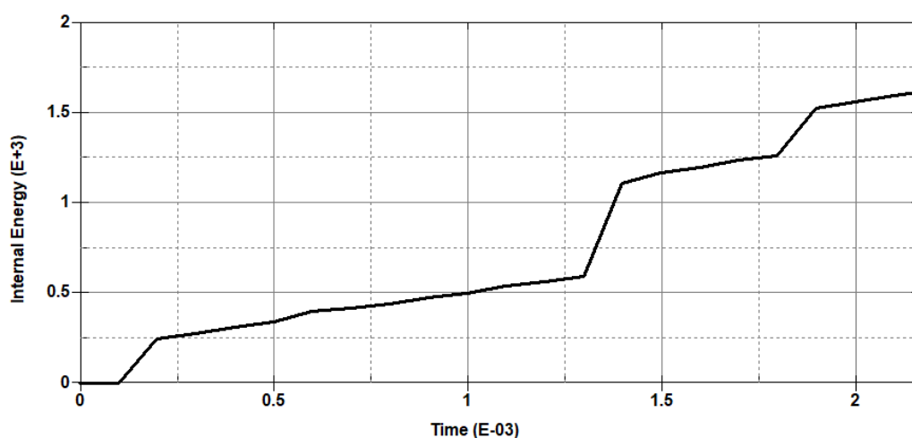
Рис.4. Залежність потрібної роботи різання від часу
