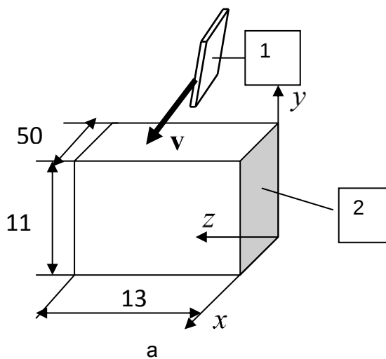
Рис.1. Схема (а) та дискретизація системи (б)
