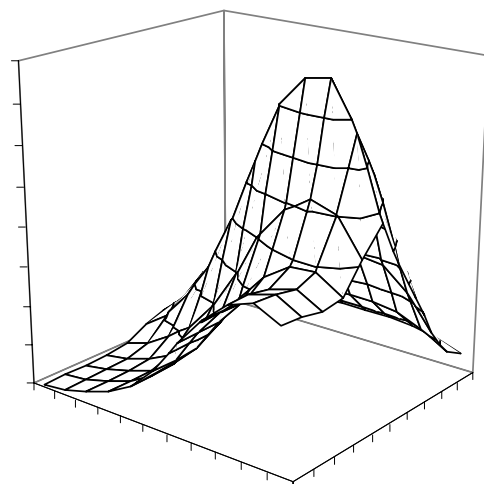
Рис. 5. Зависимость метрики IPS/A от размеров кэшей для задачи маршрутизации (RTR)
