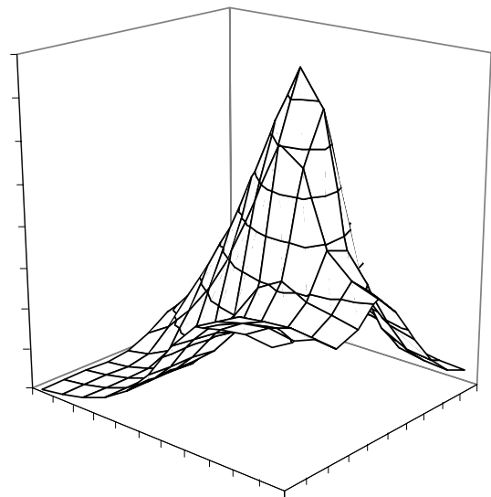
Рис. 7. Зависимость метрики IPS/A от размеров кэшей для задачи дешифровки данных (CAST)
