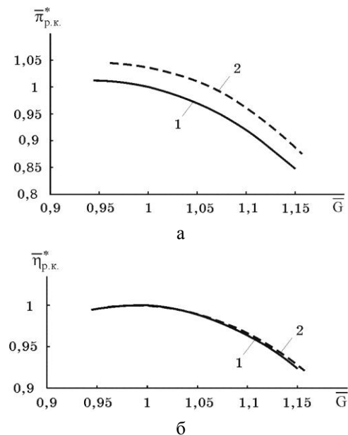
Рис. 5 Енергетичні характеристики колеса при вихідній (1) та модифікованій (2) формі лопаті а – залежність ступеня стиску і б – адіабатичного ККД від витрати повітря
