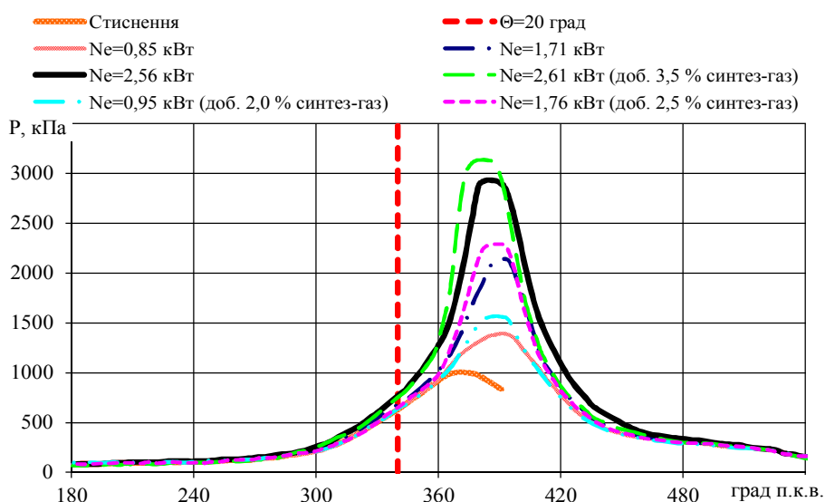
Рис. 4. Порівняння експериментальних індикаторних діаграм двигуна ІЧ 6,8/5,4 при роботі на чистому етанолі і з добавками синтез-газу
