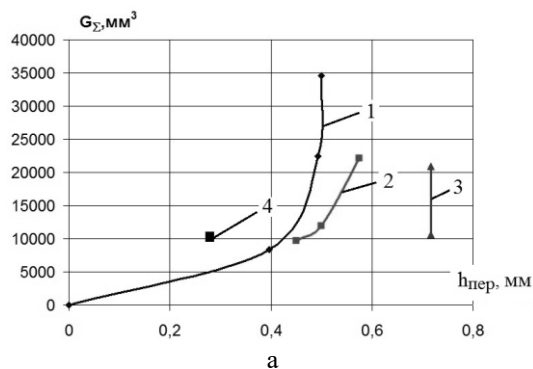
Рис. 2. Изменение снимаемого объема материала за время работы РИ (Сандвик Коромант – H13, с покрытием 0,18 HfN + 0,8 ZrN) от износа по передней (а) и задней (б) поверхности при точении закаленной стали 45 (режимы резания: 1 – V = 2,54 - 2,58 м/с, t = 0,35 мм, S = 0,15 мм/об; 2 – V = 3,38 - 3,44 м/с, t = 0,35 мм, S = 0,15 мм/об; 3 – V = 836,8 - 822,4 мм/с, t = 0,35 мм, S = 0,15 мм/об; 4 – V = 821 - 805 мм/с, S = 0,12 мм/об)
