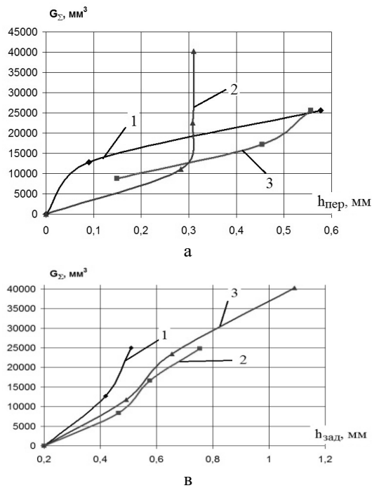
Рис. 1. Изменение снимаемого объема материала за время работы РИ (СК) с покрытием 0,18 HfN + 0,8 ZrN + Al 2 O 3 и комбинированным упрочнением от износа по передней (а), задней (в) и размера лунки (б) при обработке закаленной стали 45 HRC = 49
