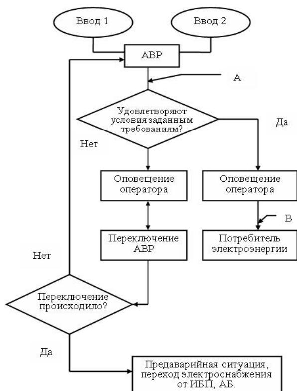
Рис. 1. Алгоритм внешней работы СККЭ А – точка контроля параметров качества на вводе системы; В – точка контроля параметров качества на вводе потребителя
