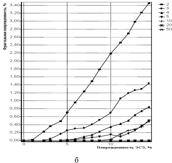
Рис. 7. Зависимость фрактальной повреждаемости при различных длинах фракталов от повреждаемости ЭСЭ: а – для количества связей n_{св} = 3 ; б – для количества связей n_{св} = 4
