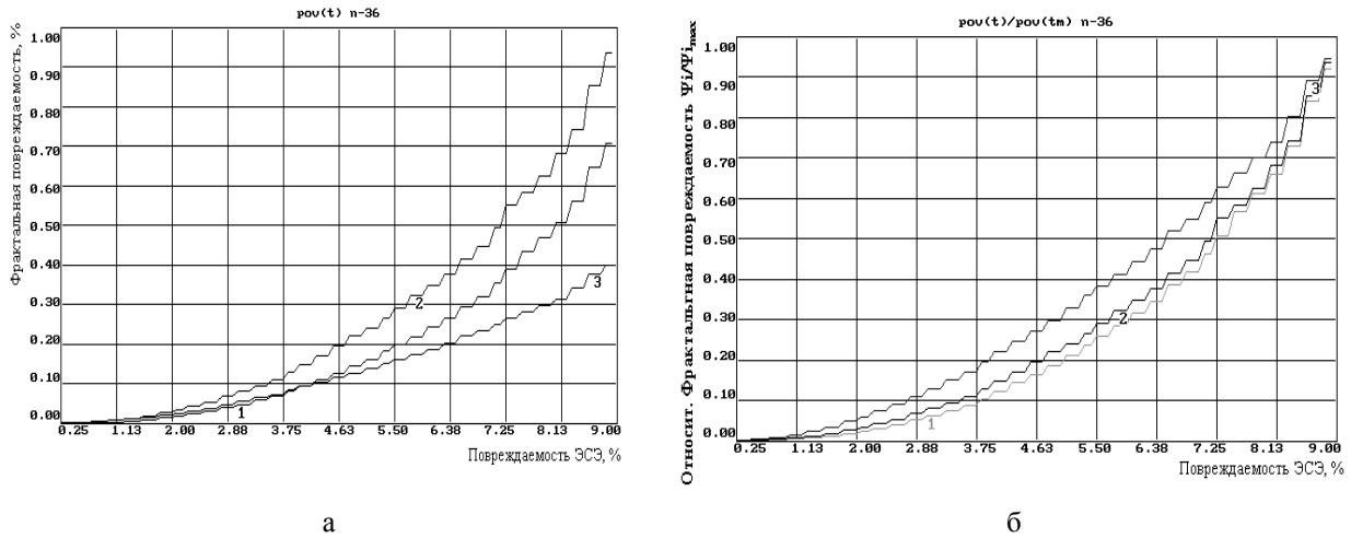
Рис. 9. Зависимость фрактальных повреждаемостей \psi_{ф\_np}(1) , \psi_{ф\_кр}(2) , \psi_{ф\_се}(3) (рис.9.а) и относительной фрактальной повреждаемости \psi_i/\psi_{max} (рис.9.б) от повреждаемости ЭСЭ (%) для n_{св} = 36
