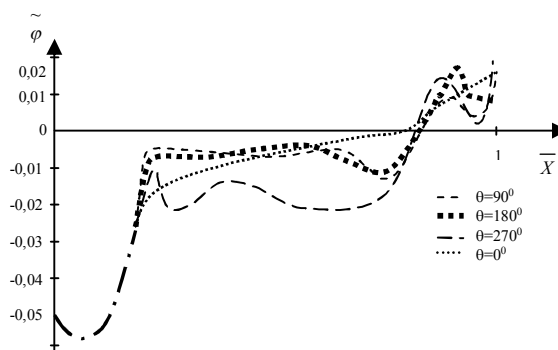
Рис. 2. Распределение потенциала по поверхности тела вращения, полученное при решении СЛАУ методом сопряженных градиентов
