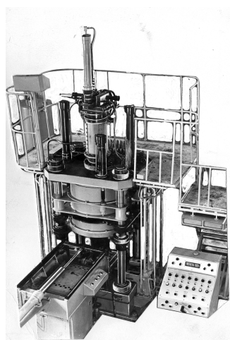
Рис. 4. Пресс-пушка ПП11М
