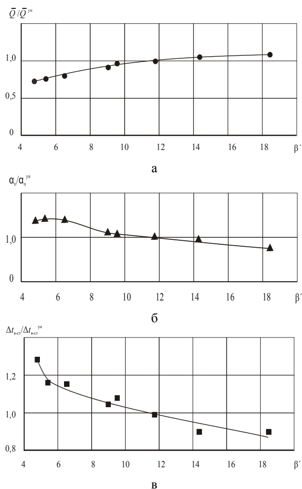
Рис. 2. Относительная тепловая нагрузка Q/Q^{ун} (а), коэффициент теплоотдачи \alpha_n/\alpha_n^{ун} (б) и разность температур \Delta t_{\theta-ct}/\Delta t_{\theta-ct}^{ун} в зависимости от коэффициента оребрения \beta' при скорости набегающего потока воздуха w_e = 2 м/с
