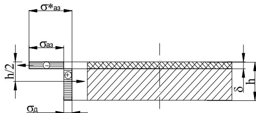
Рис. 3. Диаметрально сечение пластины
