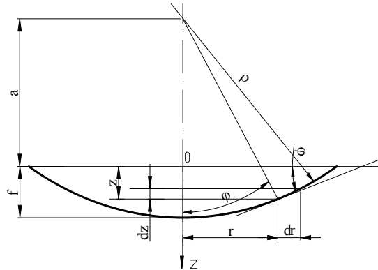
Рис. 2. Нахождение прогиба и радиуса кривизны
