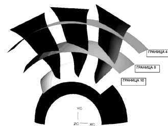
Рис. 12. Модель колеса с технологическими границами по высоте лопатки
