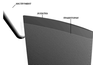
Рис. 13. Формообразование пера лопатки моноколеса спиральным высокоскоростным фрезерованием
