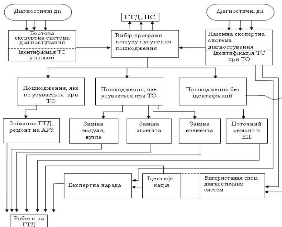
Рис. 3. Схема використання ЕС діагностування в процесі ТО ГТД (ІІ етап діагностування ГТД)
