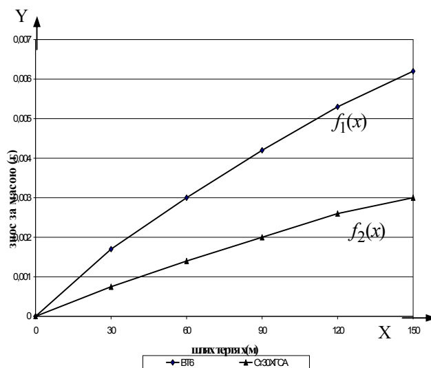
Рис. 2. Експериментальні залежності абразивного зносу за масою поверхонь матеріалів від величини шляху тертя для наступних матеріалів:
