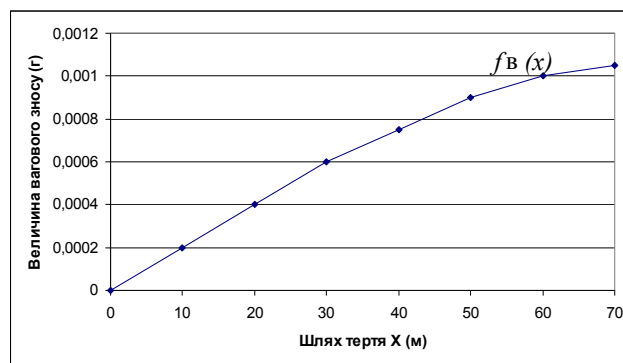
Рис. 4. Залежність величини зношування від шляху тертя боридного покриття в абразивному середовищі \text{SiO}_2 (пісок) із зернистістю 160 – 200 мкм
