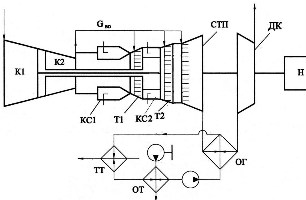
Рис. 1. Схема ГТД с промподогревом газа и силовой турбиной перерасширения: К1 и К2 – компрессоры; КС1 – основная камера сгорания; КС2 – камера сгорания промподогрева; Т1 и Т2 – турбины; СТП – силовая турбина перерасширения; ДК – дожимающий компрессор; ОГ – охладитель газа; Н – нагрузка
