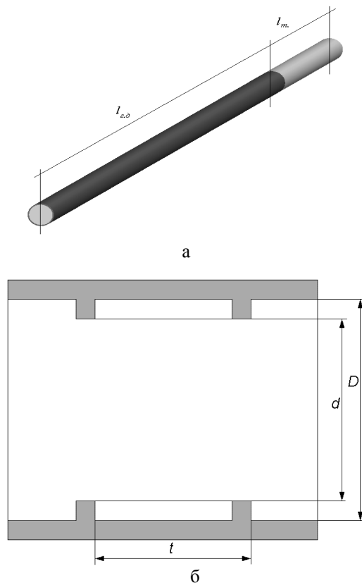
Рис. 2. Геометрическая модель цилиндрического канала (а) и продольное сечение канала на участке l_m в районе соседних интенсификаторов (б)
