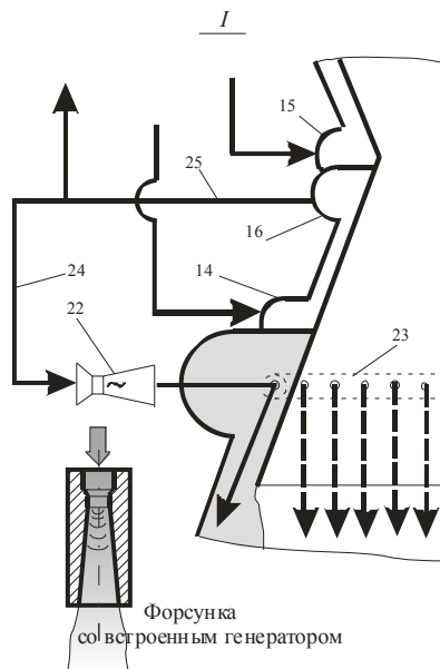
Рис. 2. Повышение полноты дожигания генераторного газа специальной форсункой
