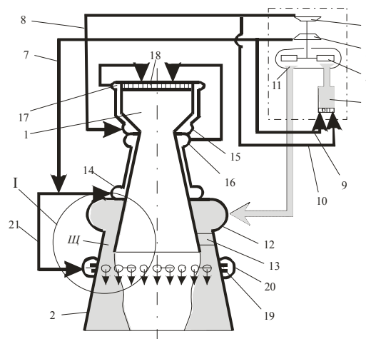
Рис. 1. Предлагаемая схема
