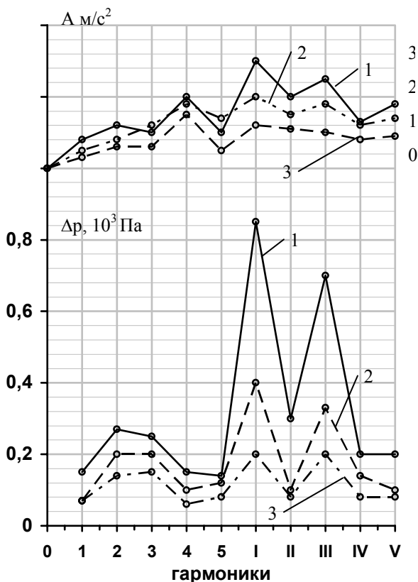
Рис. 6. Влияние радиальной длины дискового кольца на подавление пульсаций давления и вибраций корпуса насоса. 1 - D_d=0,9 D_2 , 2 - 0,8 D_2 , 3 - 0,7 D_2
